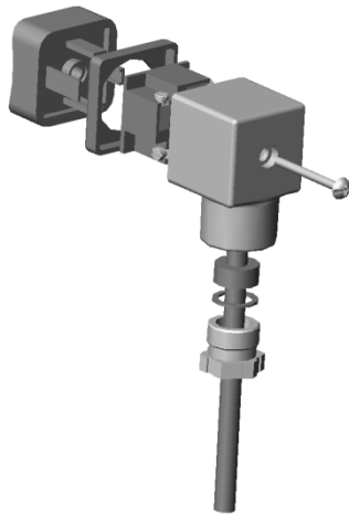
Figura 1 - Esplosi connettori
